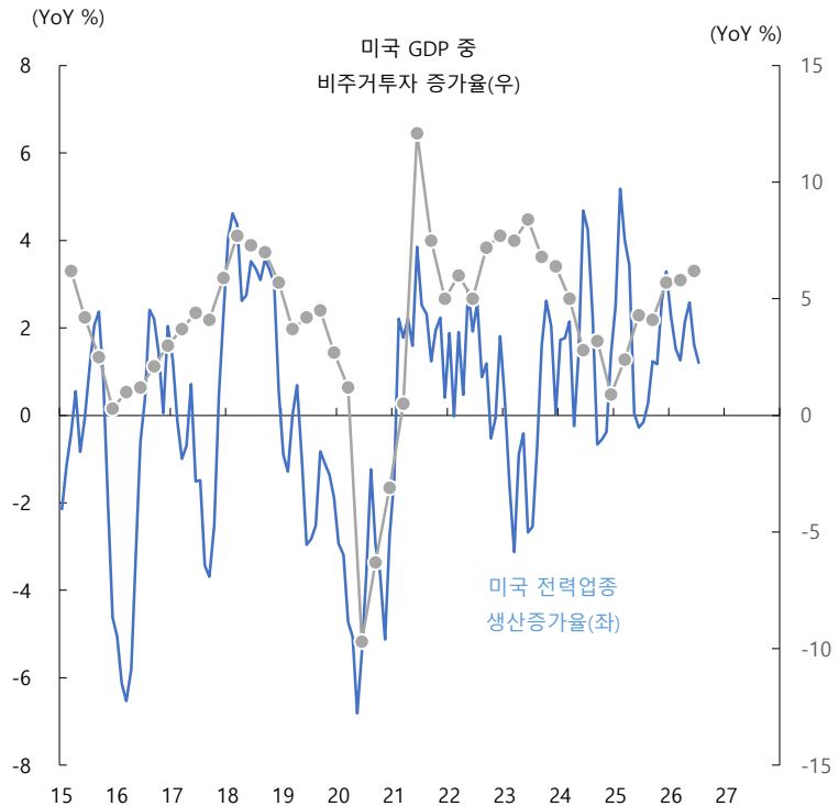
<그림> 비주거투자가 안정적인 성장 흐름을 보이고 있는 가운데 전력업종 생산도 꾸준한 증가세를 보이고 있음
